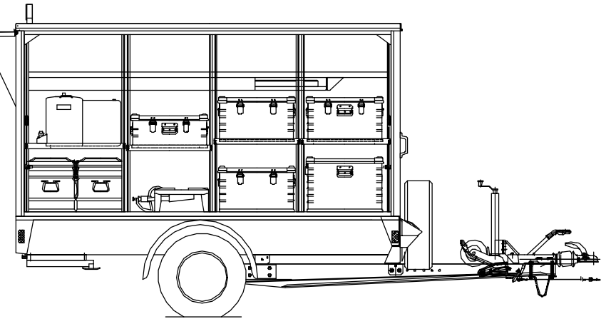
Seitenansicht rechts
