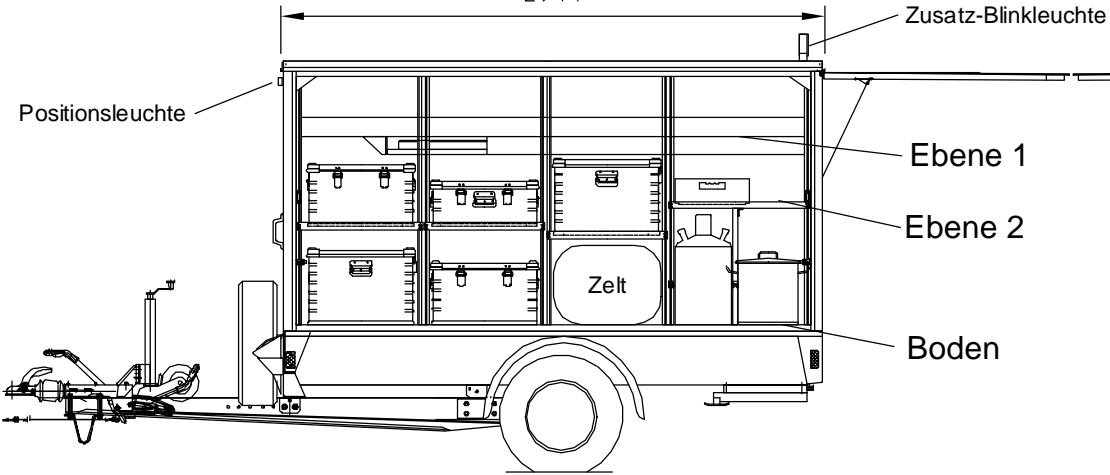
Seitenansicht links
